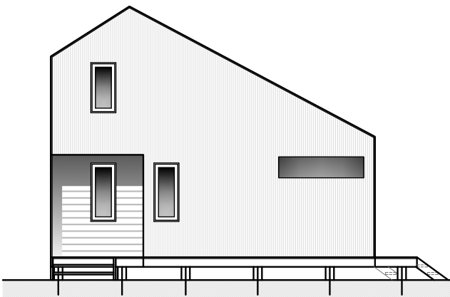
Elevacion Acceso Escala 1:50
